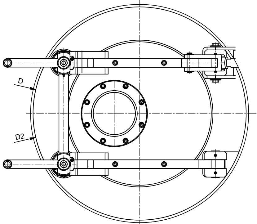
Details der Anschweissnase gemäss Kundenwunsch
