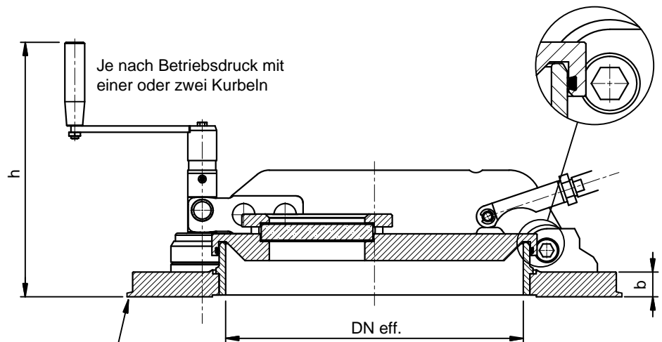
Details der Anschweissnase gemäss Kundenwunsch
